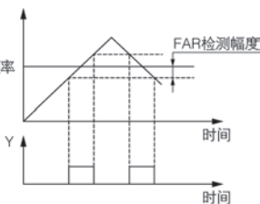
图 F7-7 频率到达示意图
