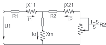
图 F2-1 异步电机稳态等效电路图
