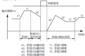
图 F9-5 PLC 启动方式 2
