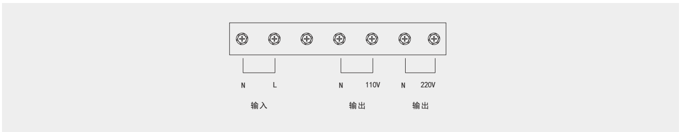
TJD-(2-3) kVA接线图
