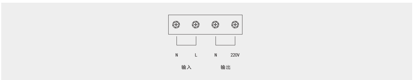
TJD-(15-30) kVA接线图
