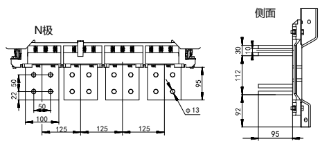
Inm=4000A水平接线尺寸
