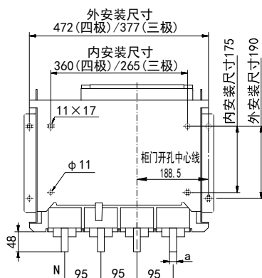
K向垂直接线及安装尺寸
