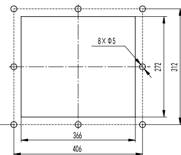
固定式柜门开孔尺寸
