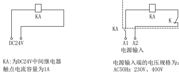
图 15 分励脱扣器控制回路设计
