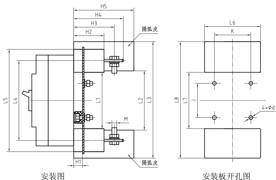
图 22 3P 插入式外形及安装尺寸
