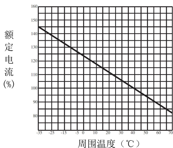
图 8 HYM3-250 温度补偿曲线
