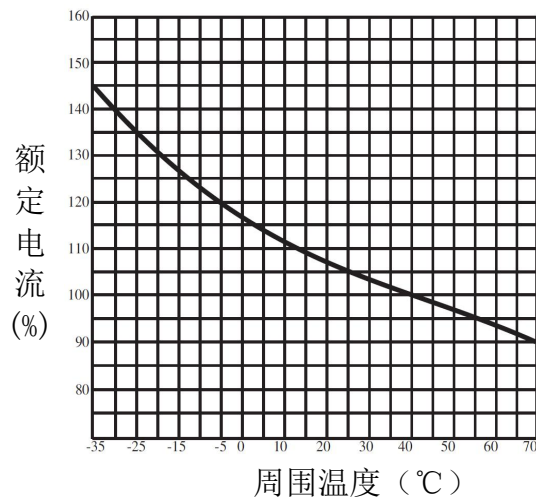
图 6 HYM3-160 温度补偿曲线
