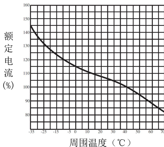
图 12 HYM3-630 温度补偿曲线
