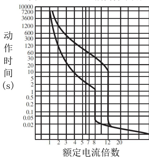
图 13 HYM3-800 动作特性曲线
