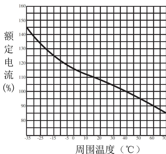
图 2 HYM3-63 温度补偿曲线
