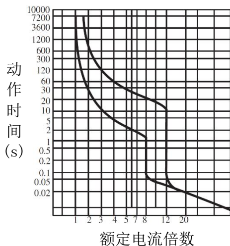
图 5 HYM3-160 动作特性曲线
