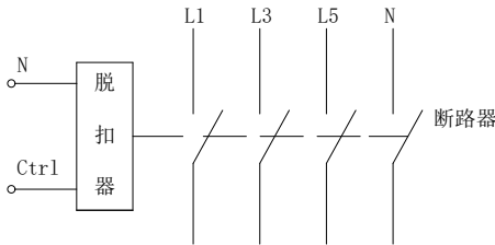
图 16 预付费电表专用脱扣器接线图
