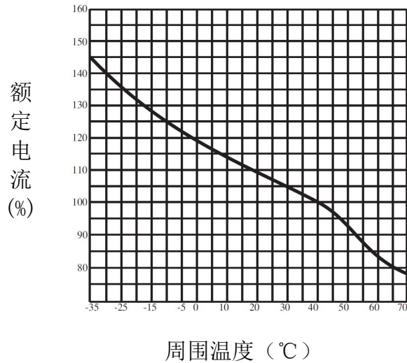
图 10 HYM3-400 温度补偿曲线
