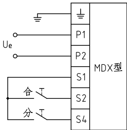
图 18 MDX 型电动操作机构的接线图
