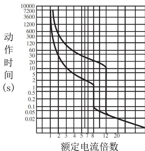
图 7 HYM3-250 动作特性曲线
