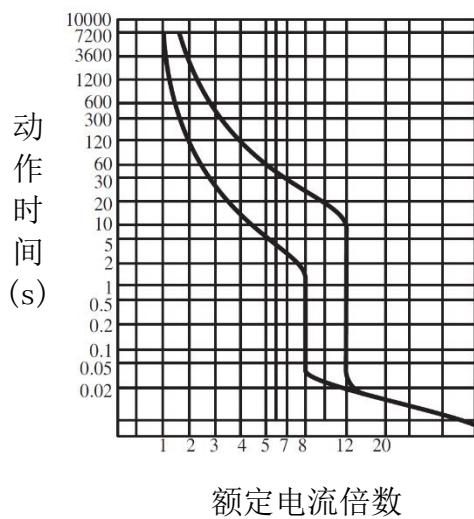
图 9 HYM3-400 动作特性曲线
