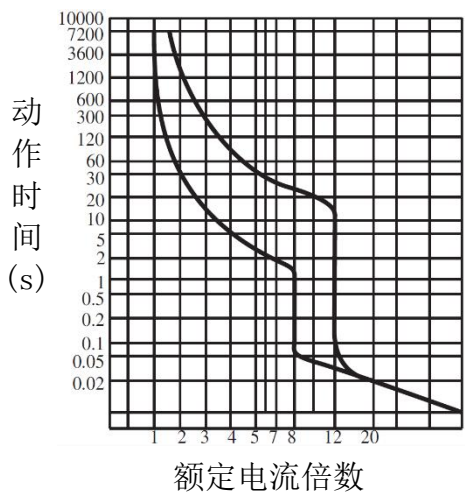
图 3 HYM3-125 动作特性曲线
