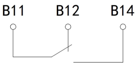
图 17 预热过载报警不脱扣接线图
