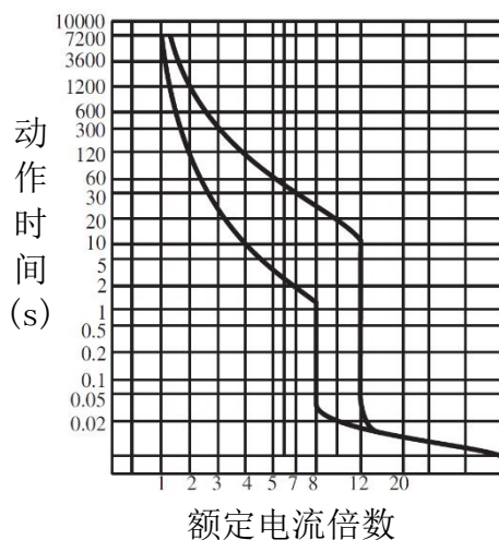
图 11 HYM3-630 动作特性曲线
