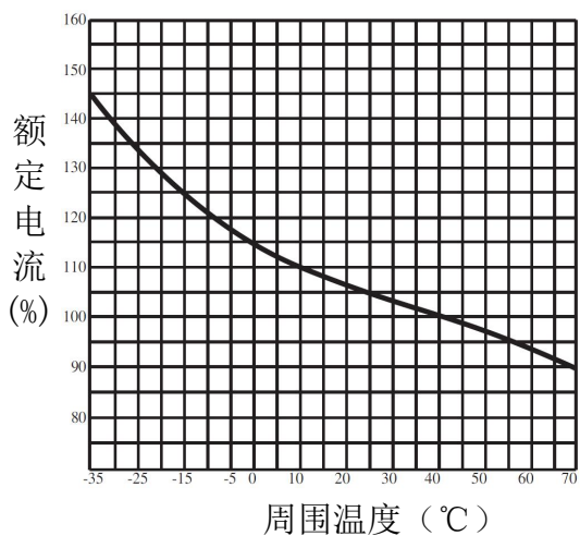
图 4 HYM3-125 温度补偿曲线
