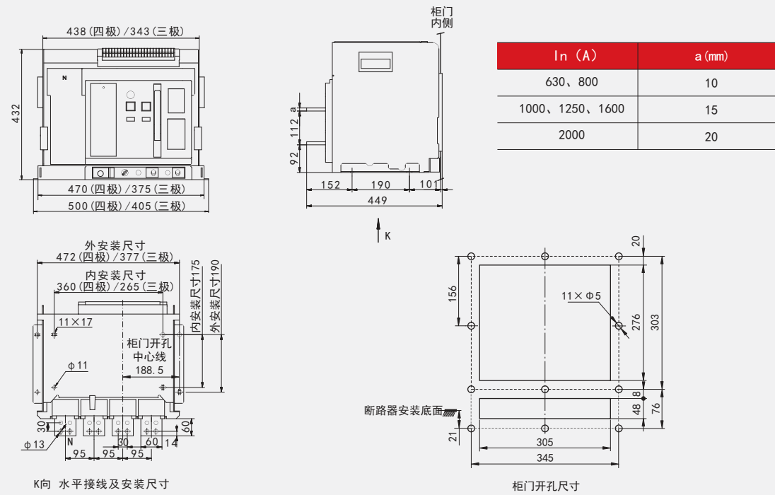
6、HUW1F-2000、HUW1PVA-2000抽屉式外形及安装尺寸
