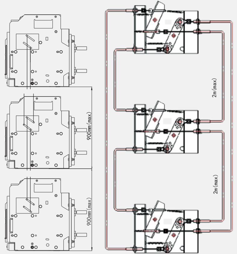
杠杆三联锁示意图
