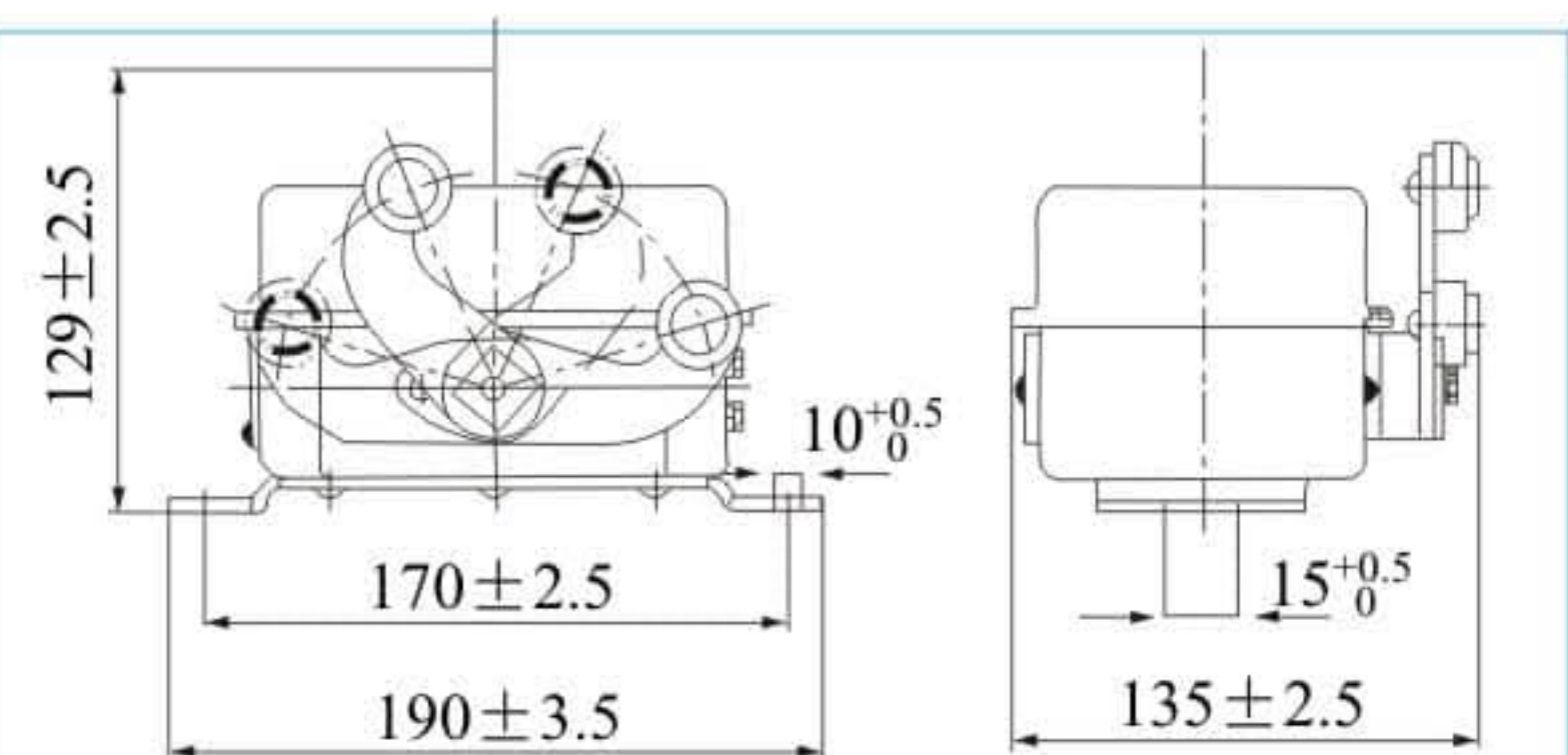
图2 LX10-21、22外形及安装尺寸
