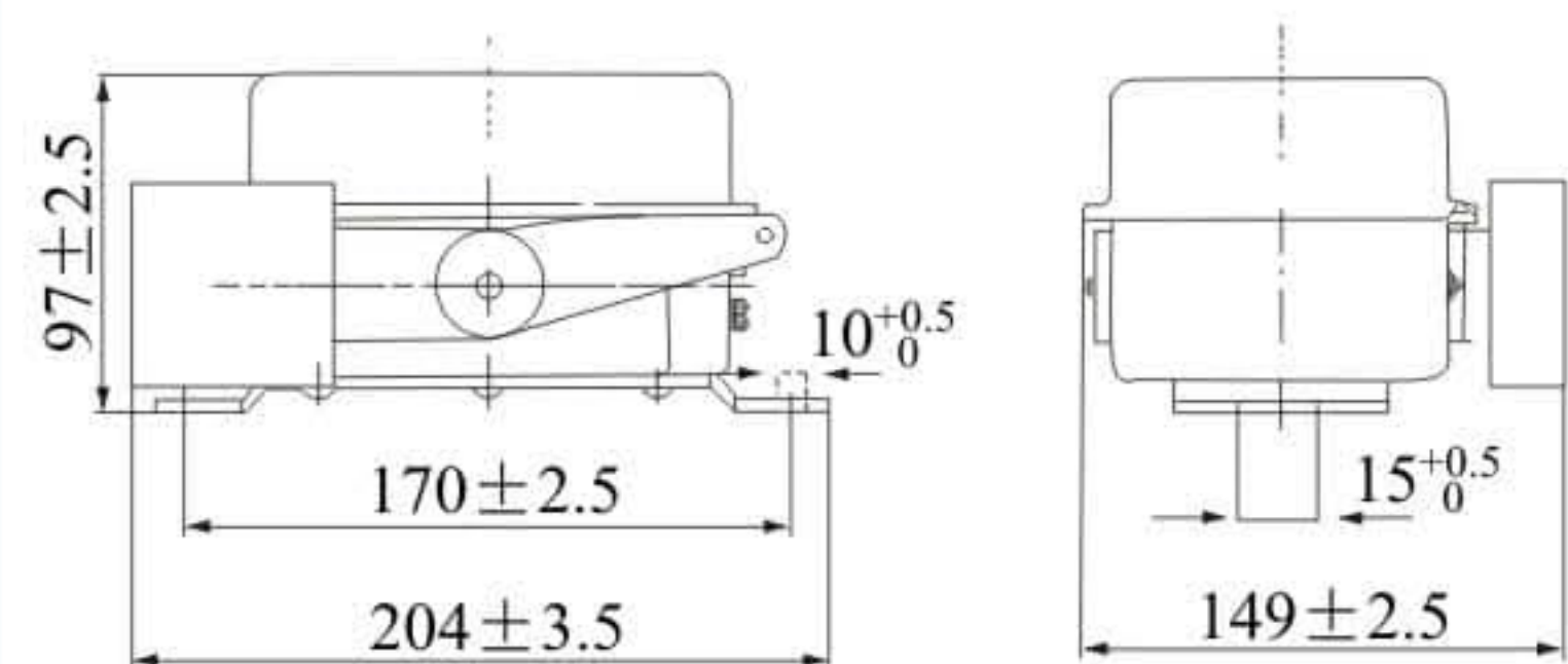
图3 LX10-31、32外形及安装尺寸
