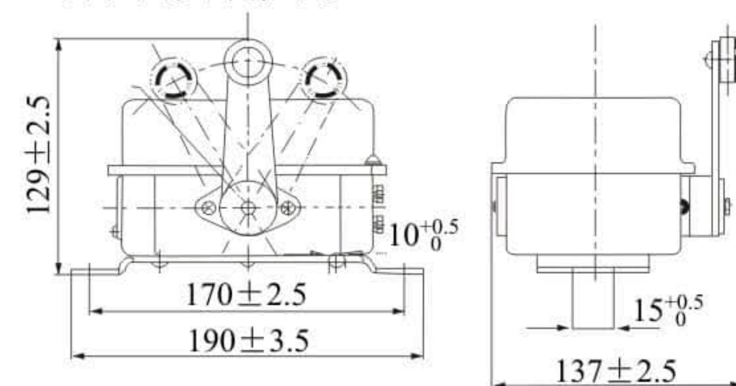
图1 LX10-11、12外形及安装尺寸
