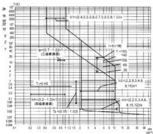
a) 短延时定时限保护特性曲线
