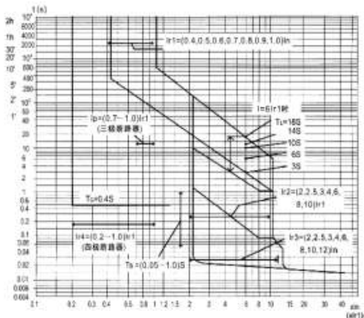
b) 短延时反时限+定时限保护特性曲线
