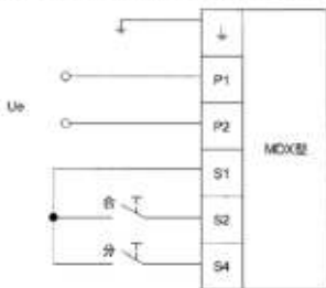
MDX 型电动操作机构接线图
