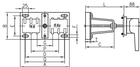
HH15S (QPS) -250 双投转换开关
