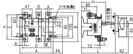
HH15P (QP) -250A
