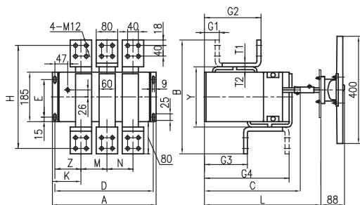
HH15P (QP) -2500、3150A
