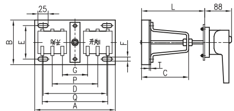
HH15S (QPS) -630~1600 双投转换开关
