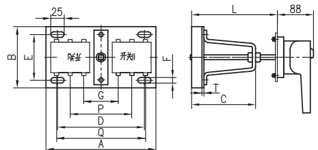
HH15S (QPS) -2500~3150、HH15 (QSS) 系列 /
