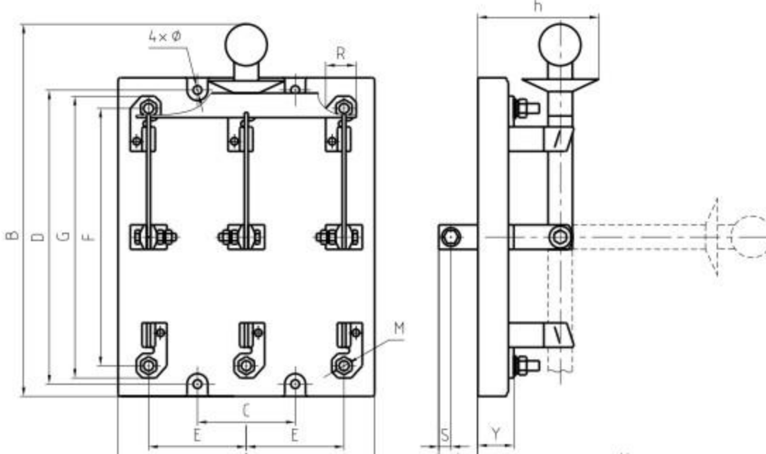
图5 HS11-200~400(板前接线板后接线)
