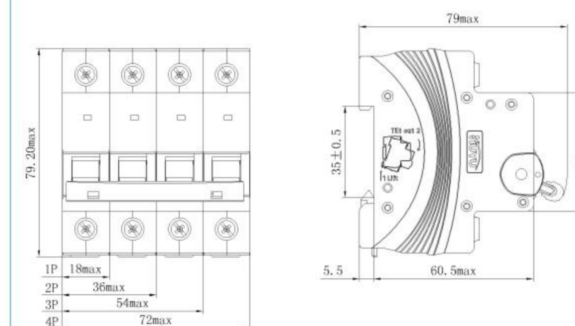
图1 外形尺寸和安装尺寸
