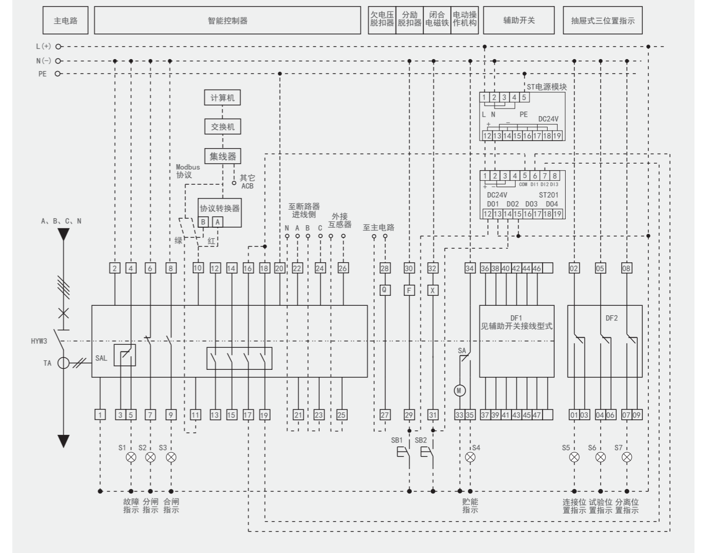
Mic5.0智能控制器二次回路接线图
