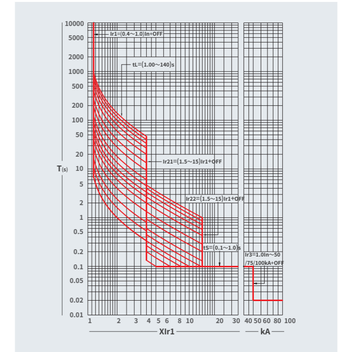
图 4、特快反时限（马达保护）
