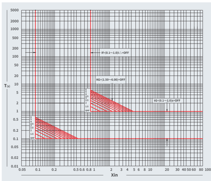
3.1、脱扣器电流整定值Ir及允差
